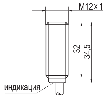
Габаритный чертеж
